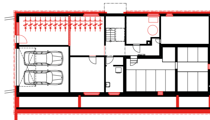
Untergeschoss
